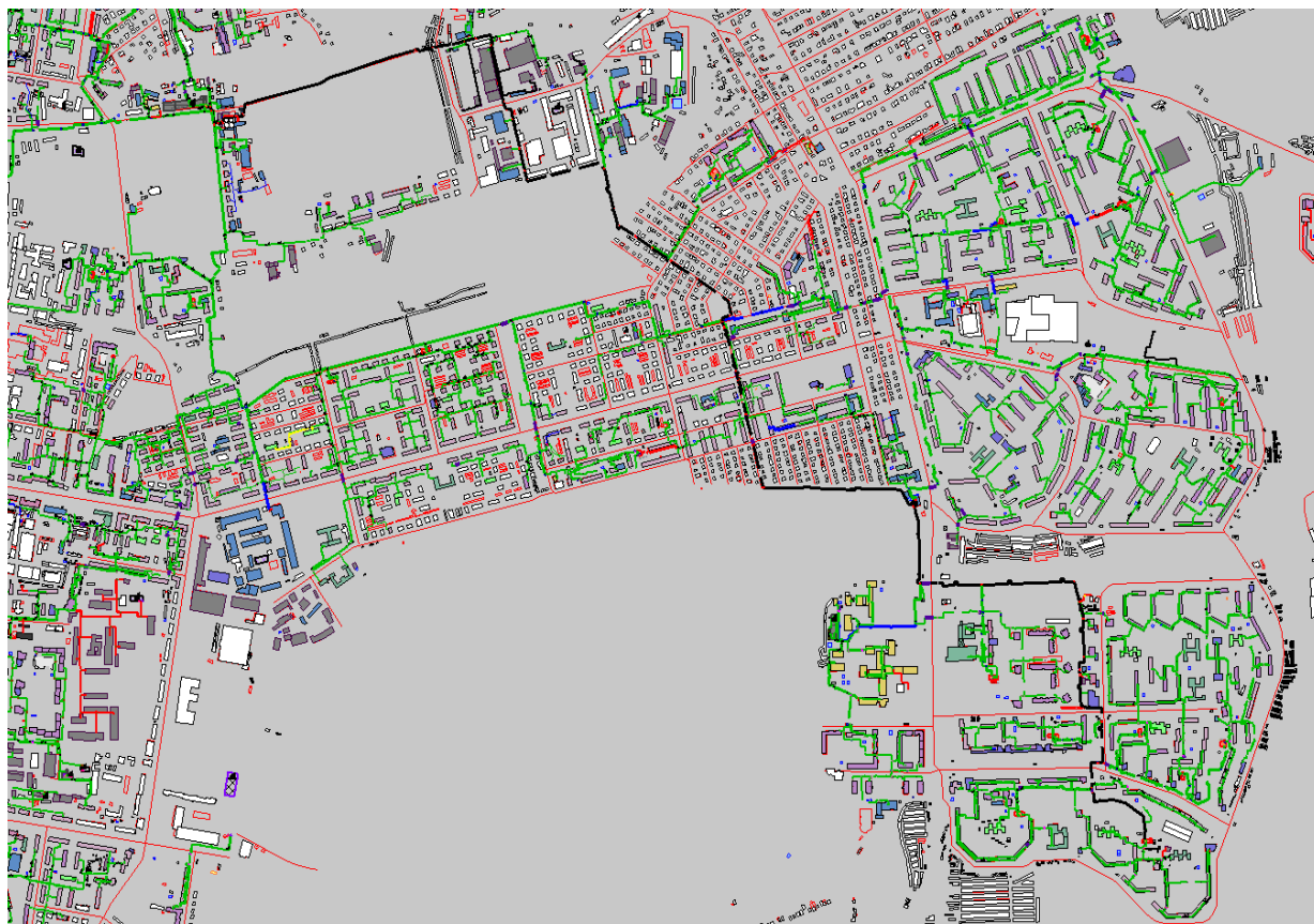
Рисунок 1.49 Результат гидравлического расчета - расчетный путь теплоносителя от котельной НТЦ до ПТ-Малин,2 пристрой
