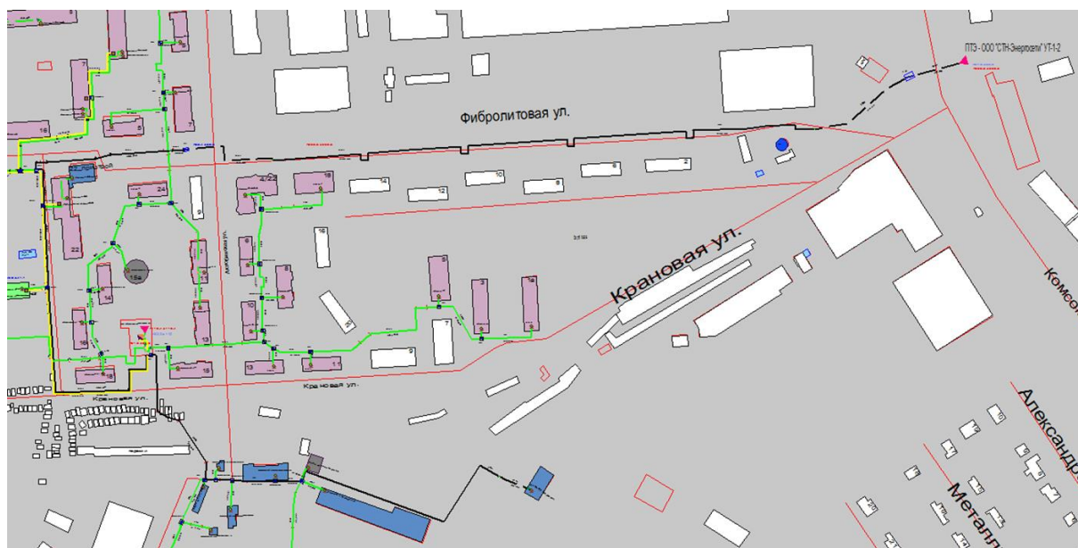
Рисунок 1.83 Результат гидравлического расчета - расчетный путь теплоносителя от котельной Московское шоссе, 62 до ПТ-Актюб.17м.
