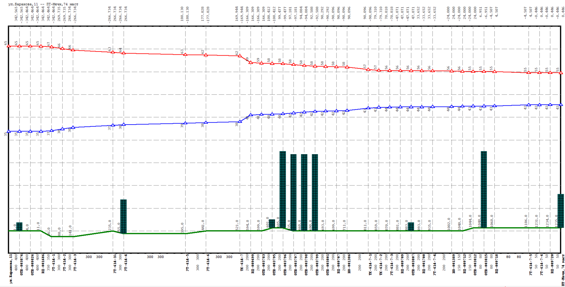
Рисунок 1.34 Результат гидравлического расчета - график гидравлических режимов по пути теплоносителя от котельной Баранова, 11 до ПТ-Меч,74 маст
