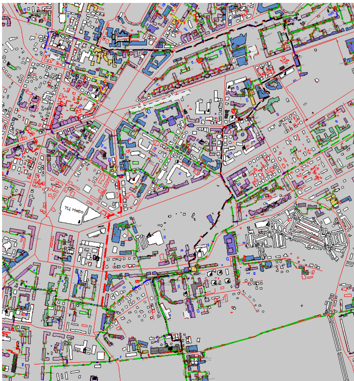
Рисунок 1.53 Результат гидравлического расчета - расчетный путь теплоносителя от котельной НТЦ до ПТ-М.Покр,7_прист.
