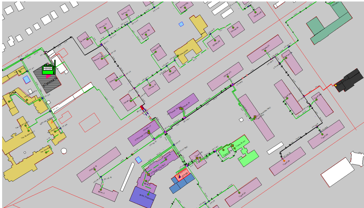
Рисунок 1.99 Результат гидравлического расчета - расчетный путь теплоносителя от котельной Таллинская, 15в до ПТ-Горох,26
