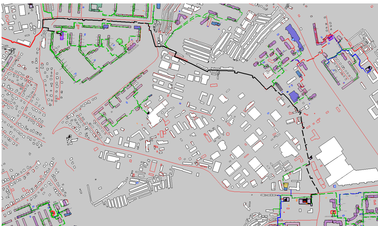
Рисунок 1.21 Результат гидравлического расчета - расчетный путь теплоносителя от котельной Деловая, 14 до ЦТП-128
