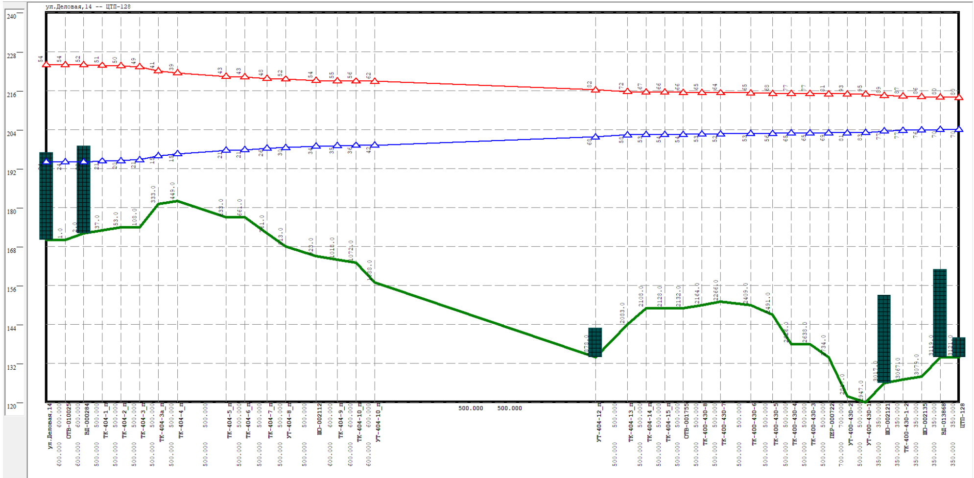
Рисунок 1.22 Результат гидравлического расчета - график гидравлических режимов по пути теплоносителя от котельной Деловая, 14 до ЦТП-128
