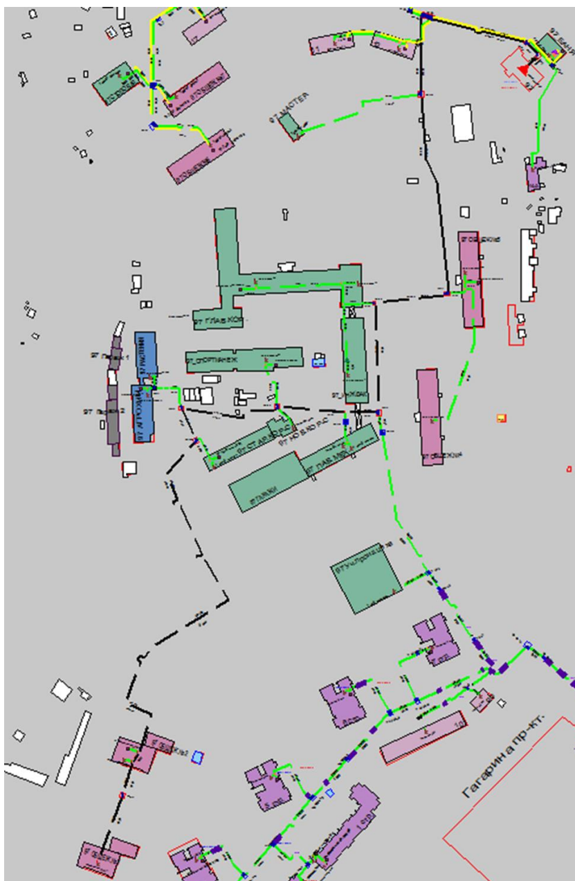
Рисунок 1.31 Результат гидравлического расчета - расчетный путь теплоносителя от котельной пр. Гагарина, 97 до ПТ-Гагар,97 общ.№1
