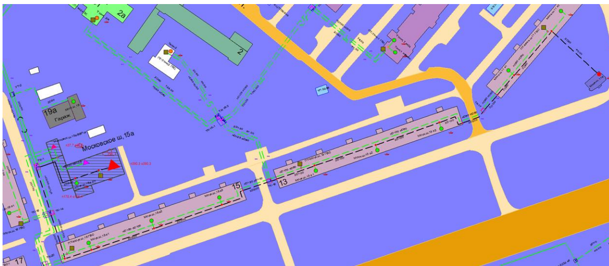
Рисунок 1.27 Результат гидравлического расчета - расчетный путь теплоносителя от котельной Московское шоссе, 15а до ПТ-Моск.ш,11а
