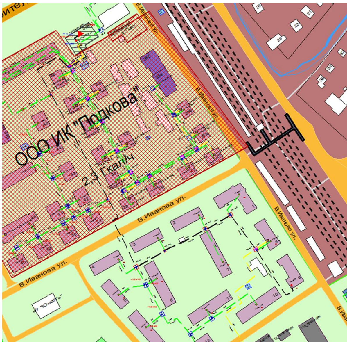
Рисунок 1.115 Расчетные пути для гидравлического расчета тепловых сетей котельной ул. Иванова, 36-б
