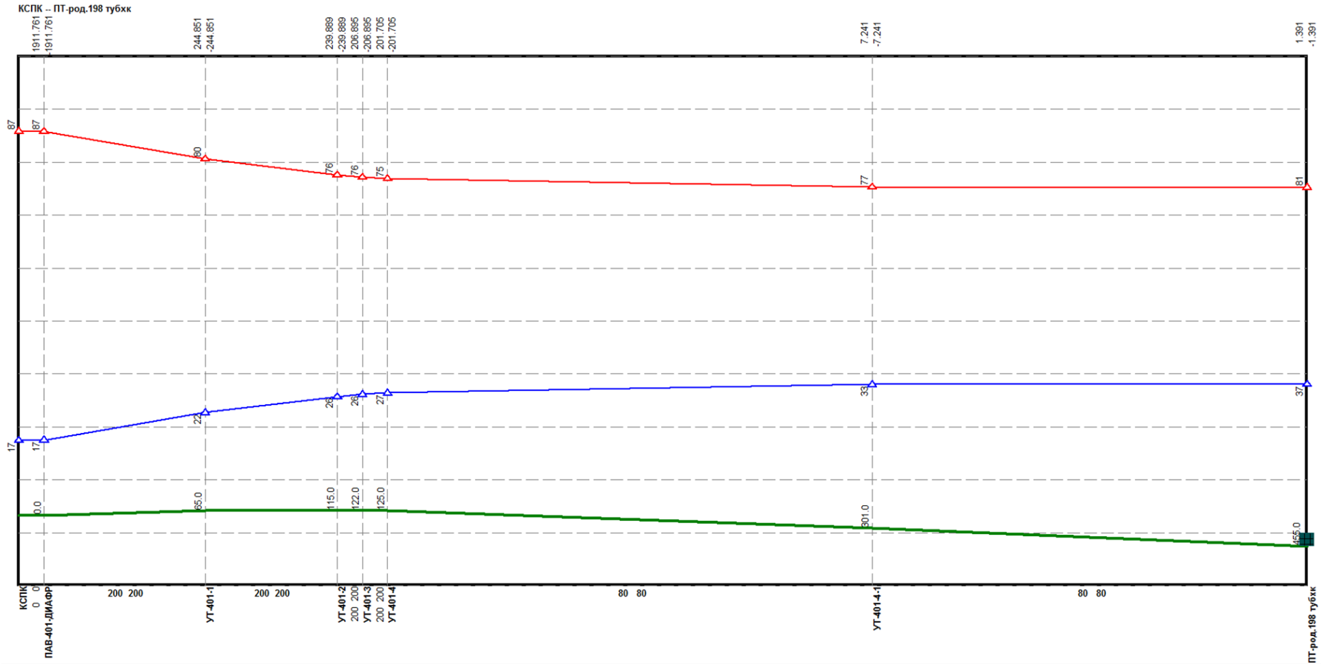
Рисунок 1.68 Результат гидравлического расчета - график гидравлических режимов по пути теплоносителя от котельной ул. Родионова, 194б до ПТ-род.198 тубкк
