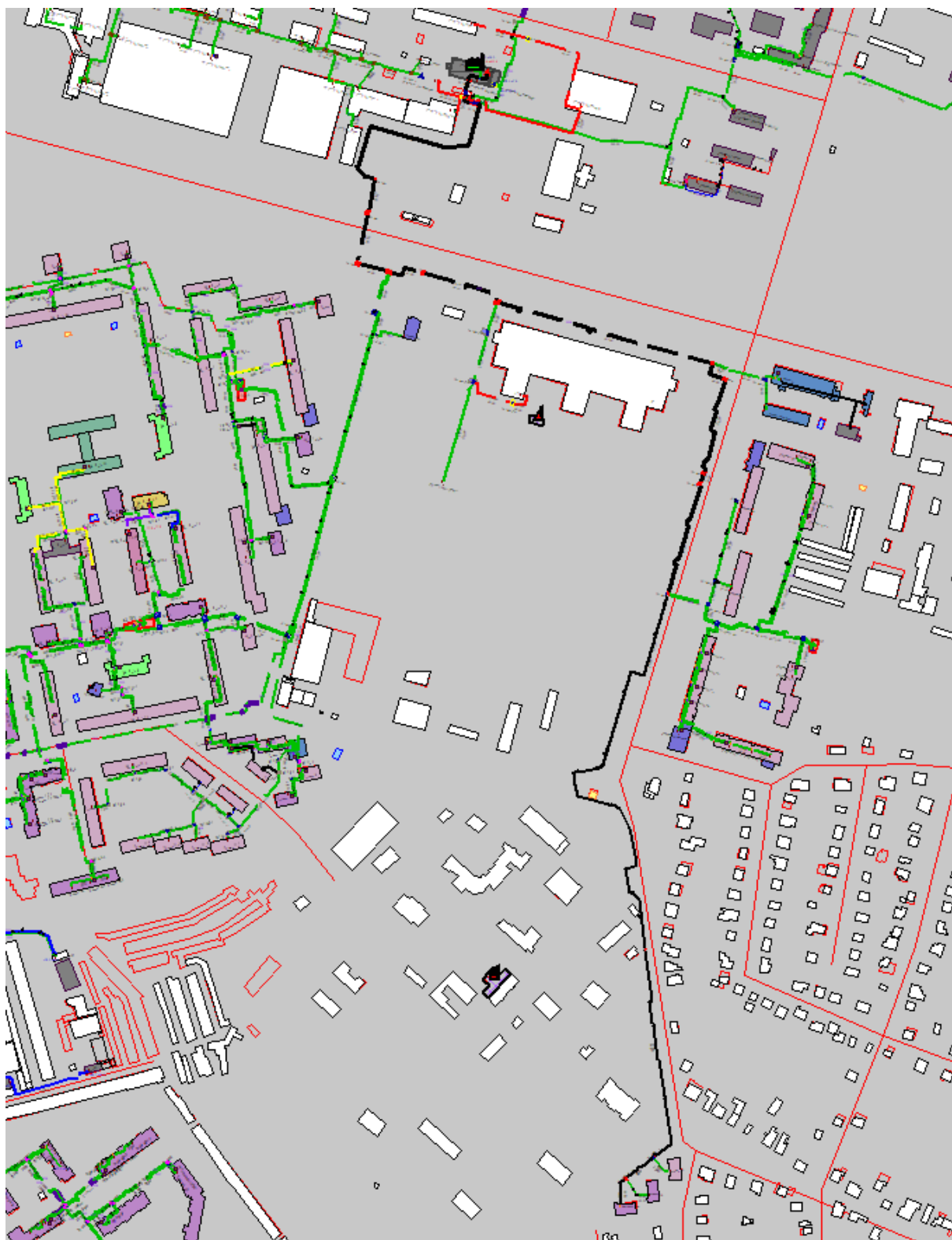
Рисунок 1.55 Результат гидравлического расчета - расчетный путь теплоносителя от котельной пр. Гагарина, 1786 до ПТ-Кашенко,14а
