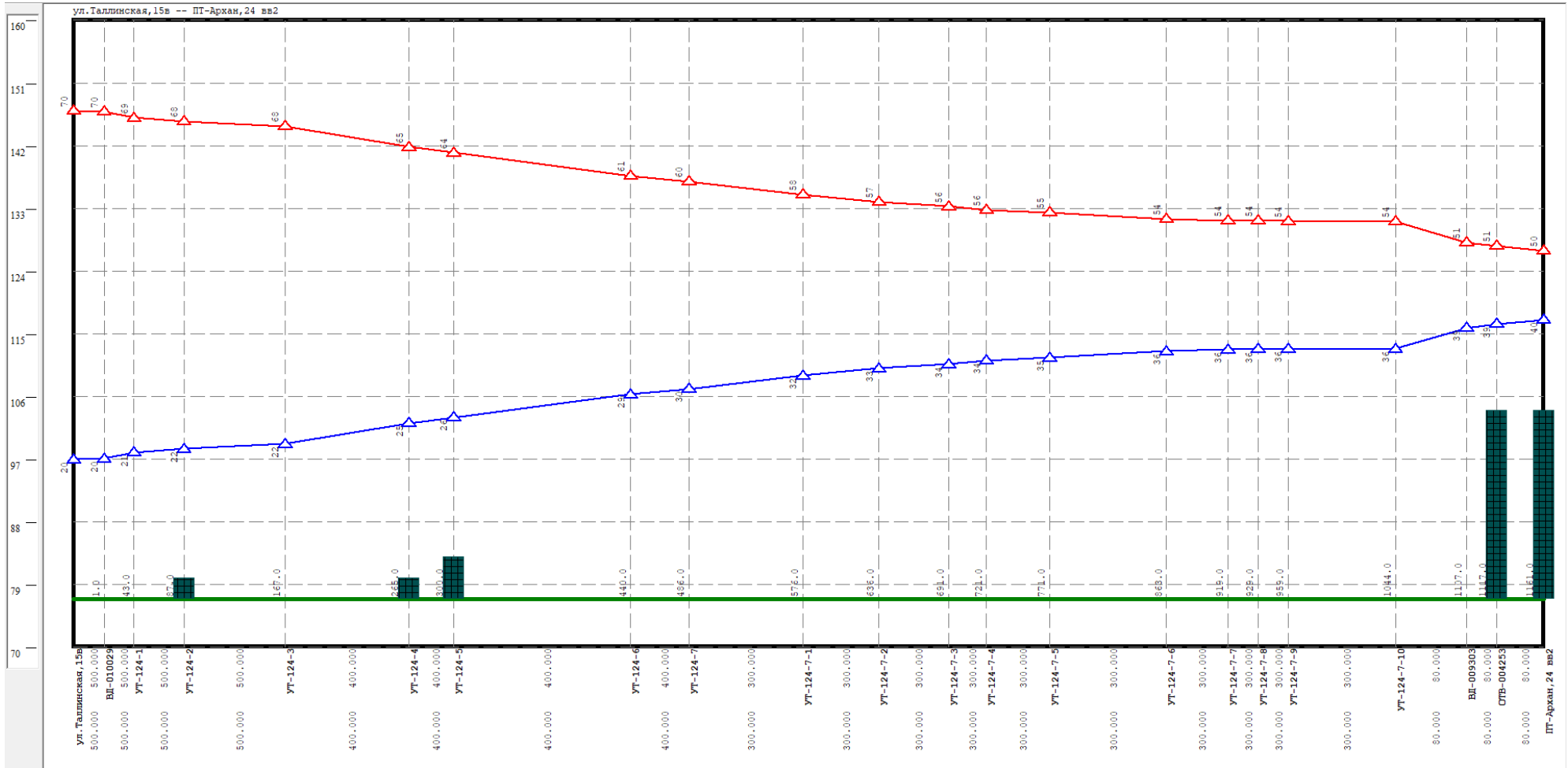
Рисунок 1.102 Результат гидравлического расчета - график гидравлических режимов по пути теплоносителя от котельной Таллинская, 15в до ПТ-Архан, 24 вв2
